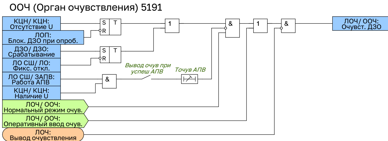
Рисунок 2.8 – Функциональная схема логики оцувствлення
