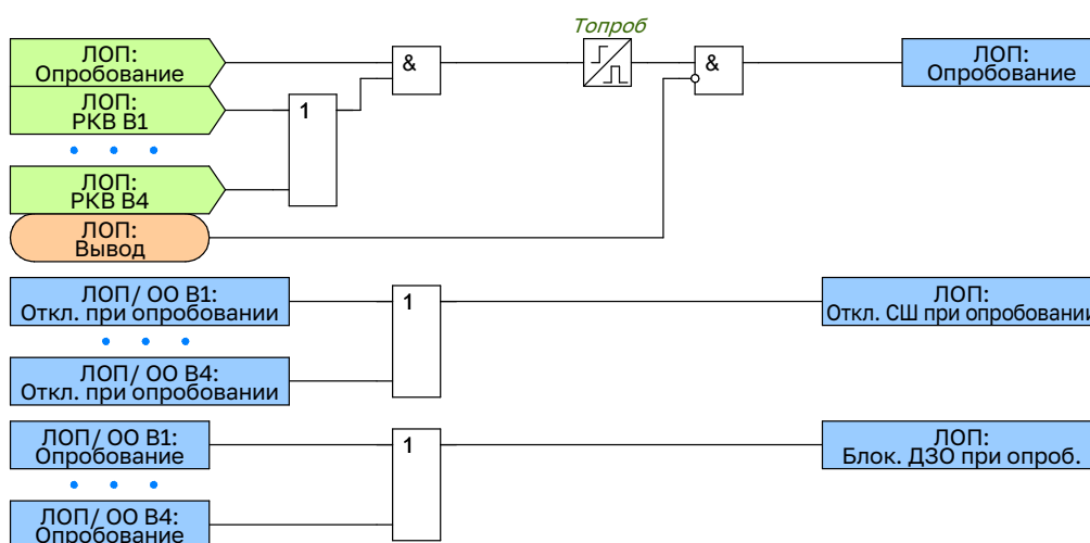
Рисунок 2.7 – Функциональная схема ЛОП
